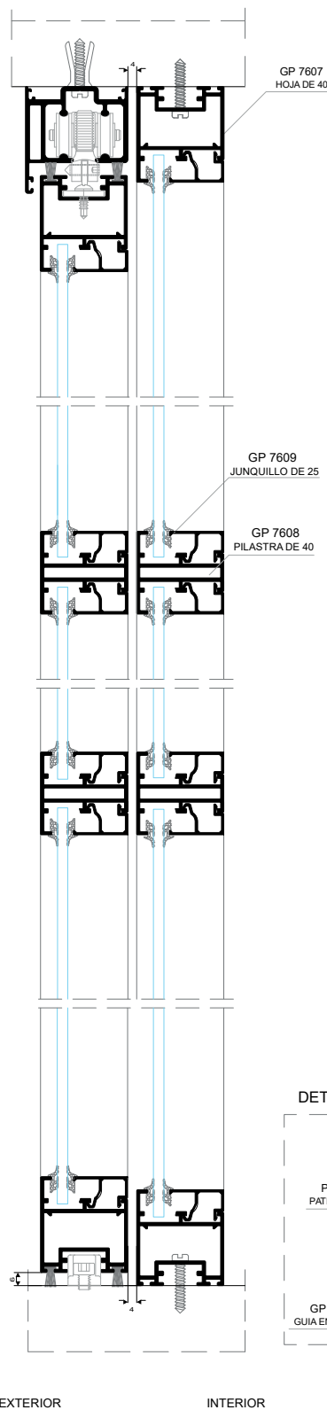
DETALLE CORREDERA + LOFT AJUNQUILLADO
