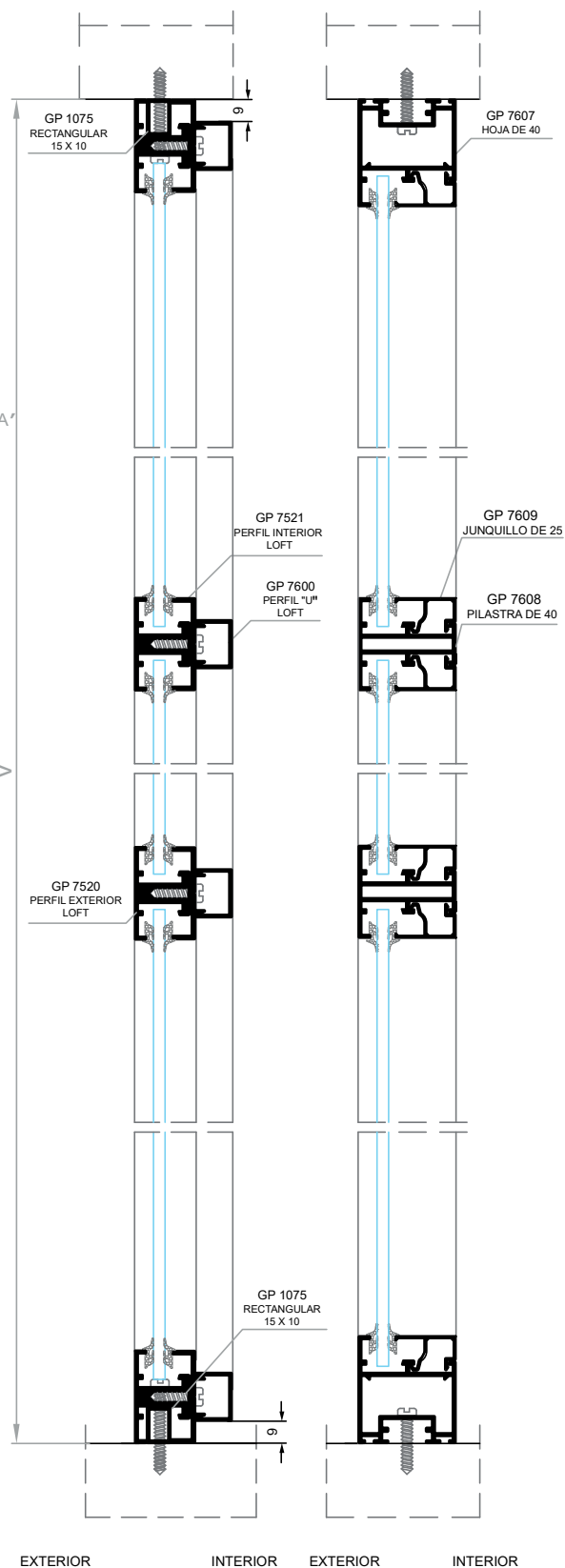
SECCIÓN VERTICAL B-B'
