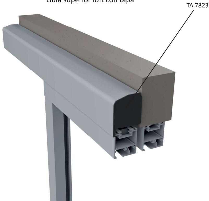
Guía superior loft con tapa
