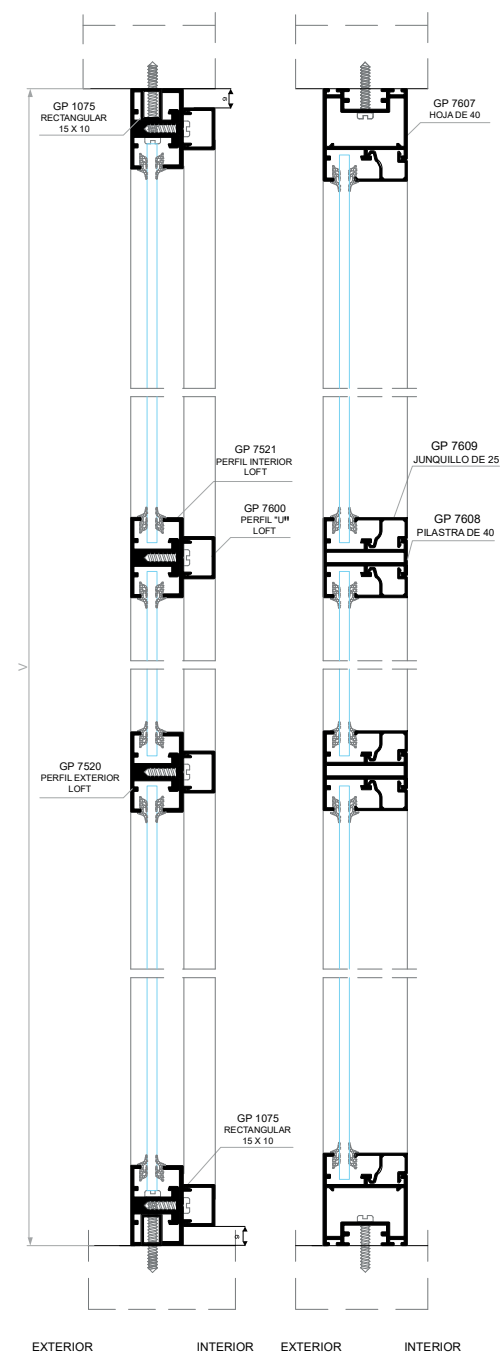
SECCIÓN VERTICAL B-B'
