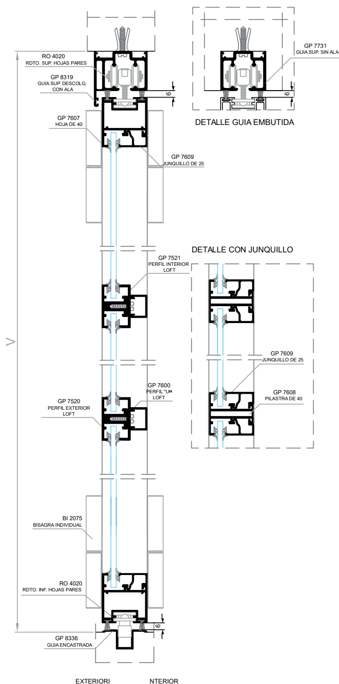
SECCIÓN VERTICAL B-B'
