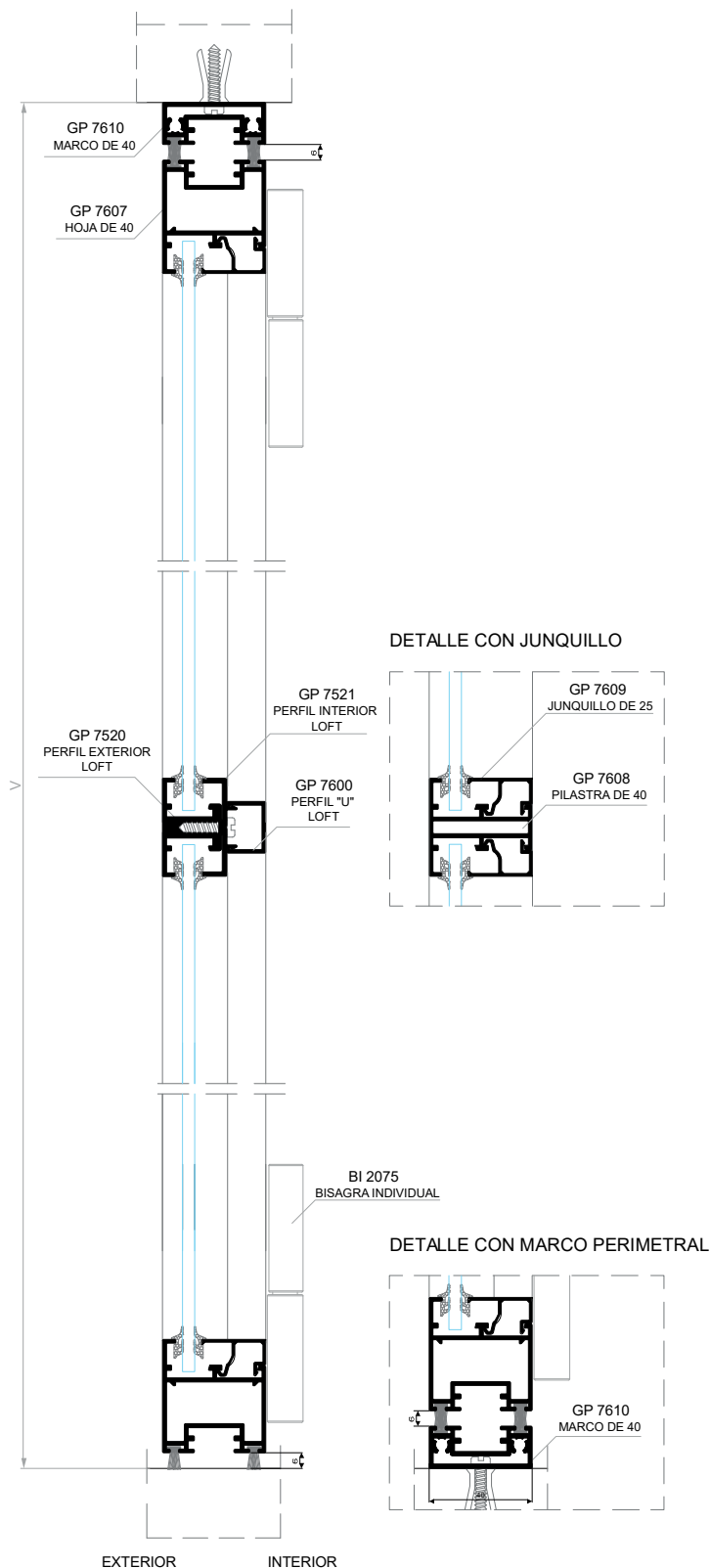
SECCIÓN VERTICAL B-B'
