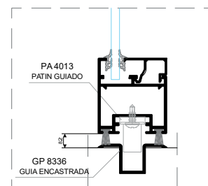
DETALLE CON GUÍA ENCASTRADA
