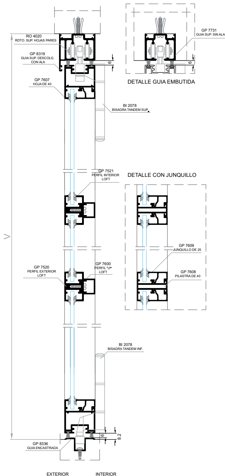
SECCIÓN VERTICAL B-B'
