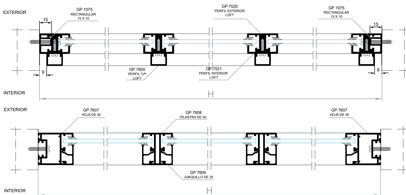
SECCIÓN HORIZONTAL A-A'
