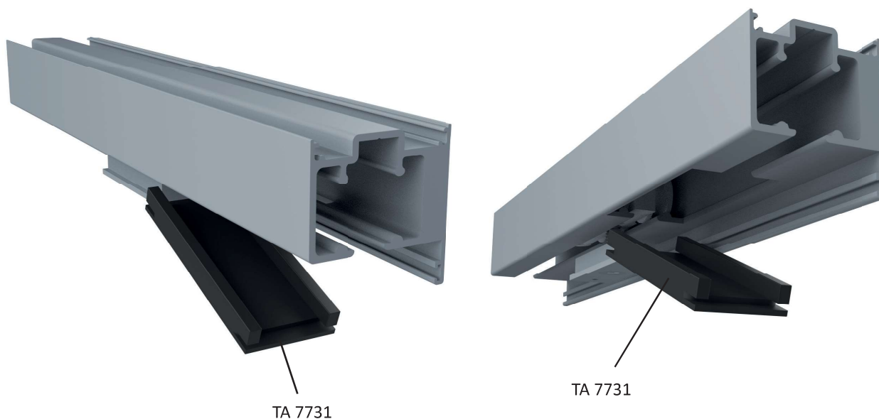
Cajeado inferior para rodamiento
