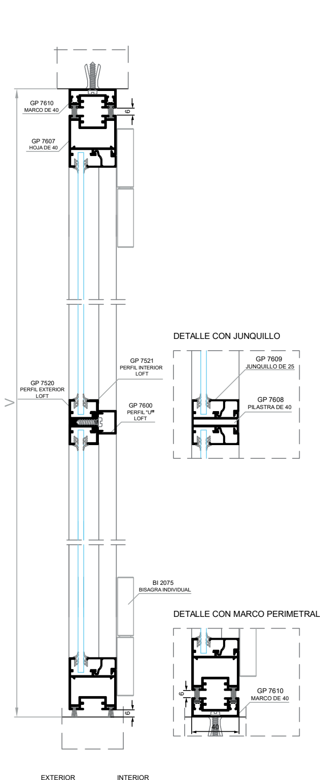
SECCIÓN VERTICAL B-B'
