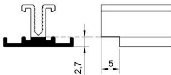
Dimensiones de corte aproximadas (mm)
