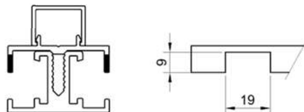
Dimensiones de corte aproximadas (mm)
